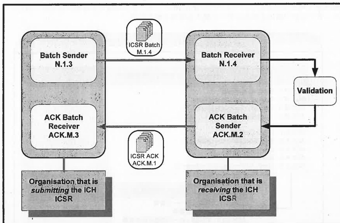
ACK.M/A ICH ICSRバッチ確認応答
