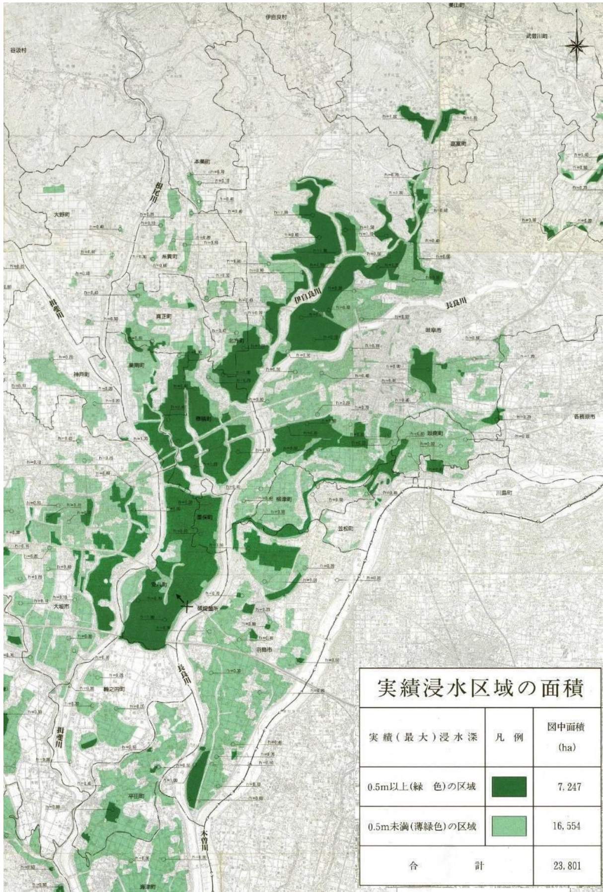
図- 1.4 昭和51年9月洪水実績図
