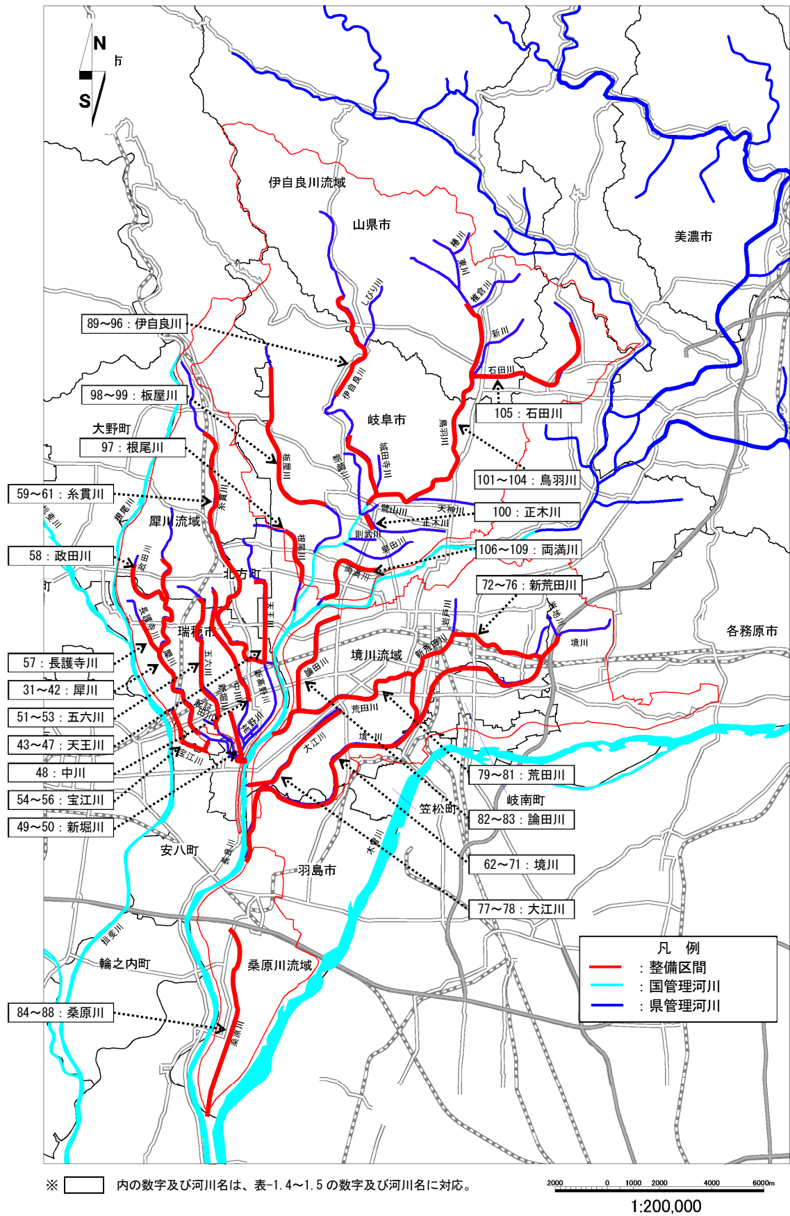
図- 1.15 長良川中流支川流域におけるこれまでの主要な河川区域内施設整備の実施箇所
