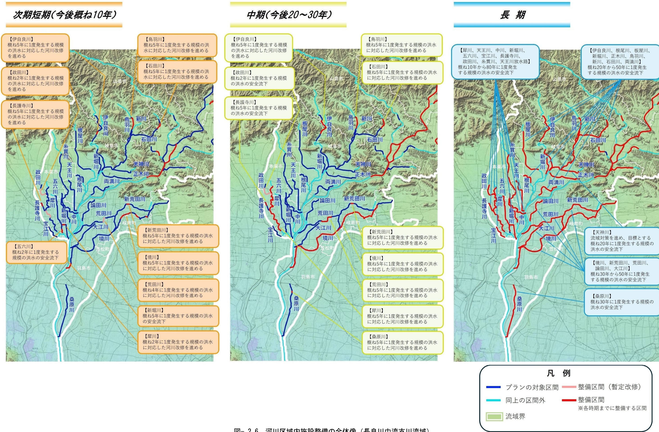
図- 2.6 河川区域内施設整備の全体像(長良川中流支川流域)
