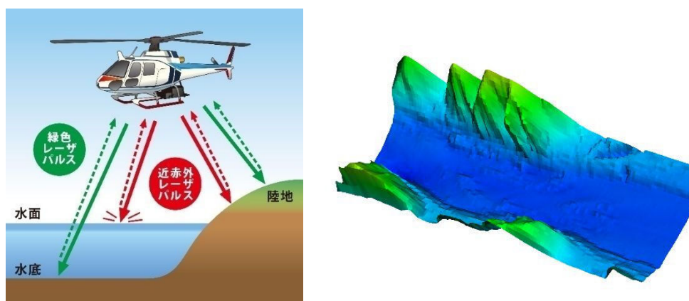
図- 2.8 航空レーザ測深（ALB）の計測イメージ河道の三次元計測データ
