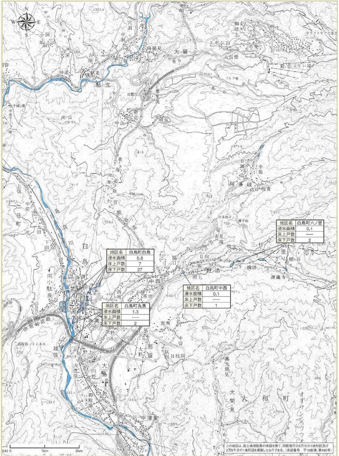
図- 1.11 平成16年10月台風第23号洪水実績図（郡上市周辺その2）
