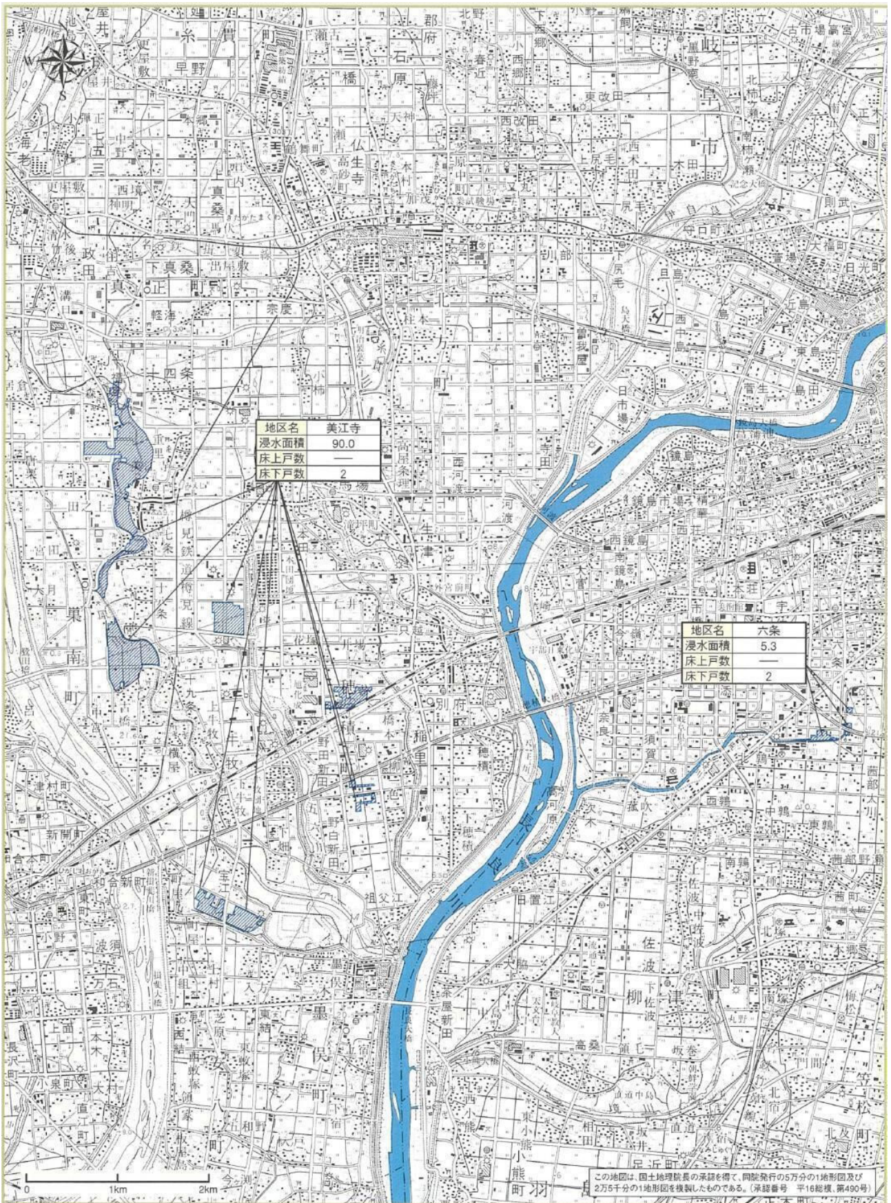
図-1.6 平成16年10月台風第23号洪水実績図（岐阜市周辺その1）
