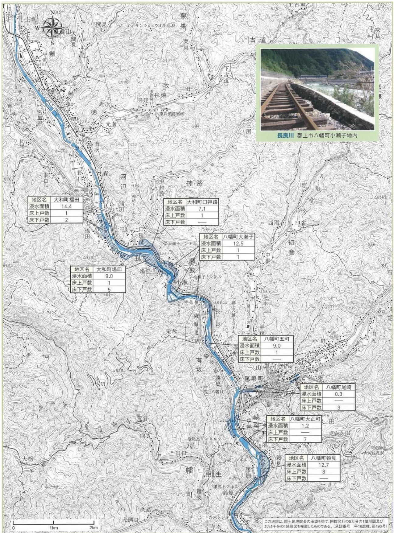
図- 1.10 平成16年10月台風第23号洪水実績図（郡上市周辺その1）
