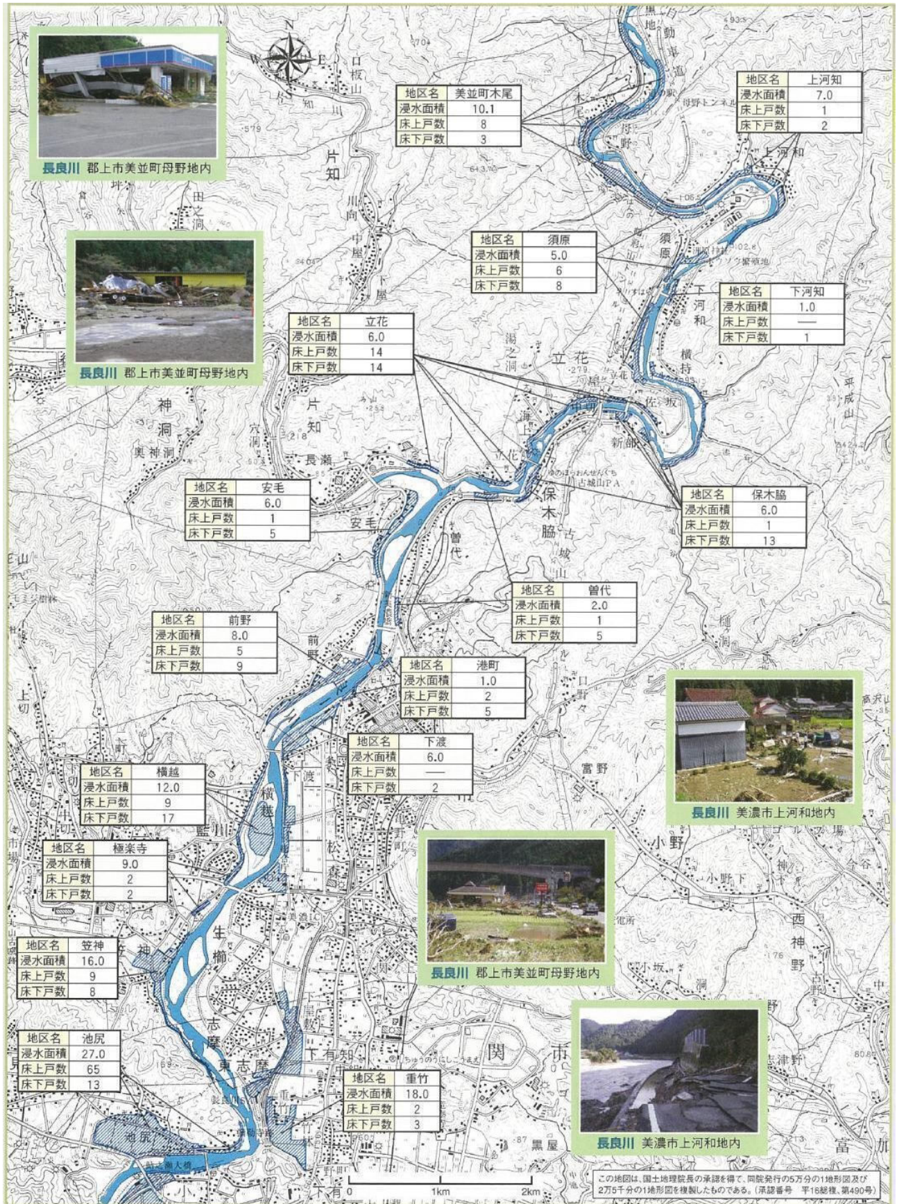
図-1.8 平成16年10月台風第23号洪水実績図（関市～美濃市周辺その1）
