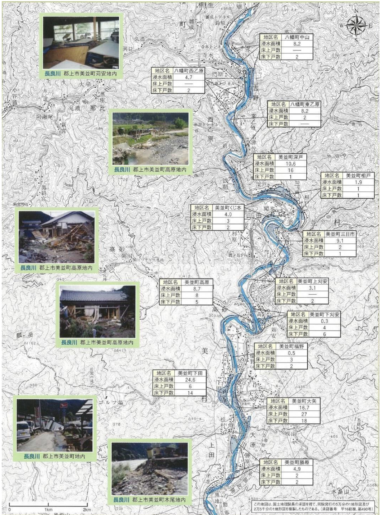
図-1.9 平成16年10月台風第23号洪水実績図（関市～美濃市周辺その2）
