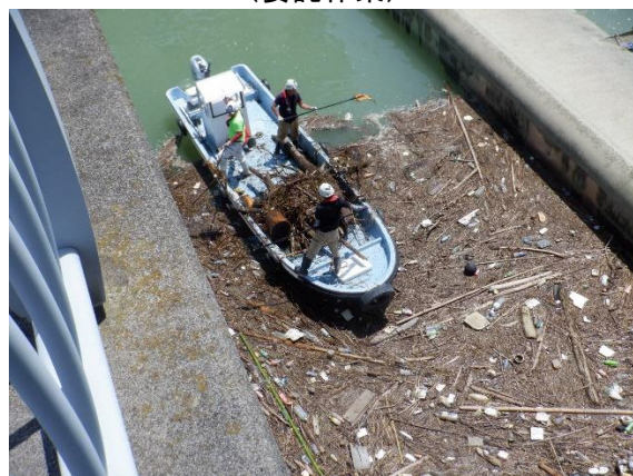
堰上流に滞留した流木等の収集引き上げ状況 (委託作業)
