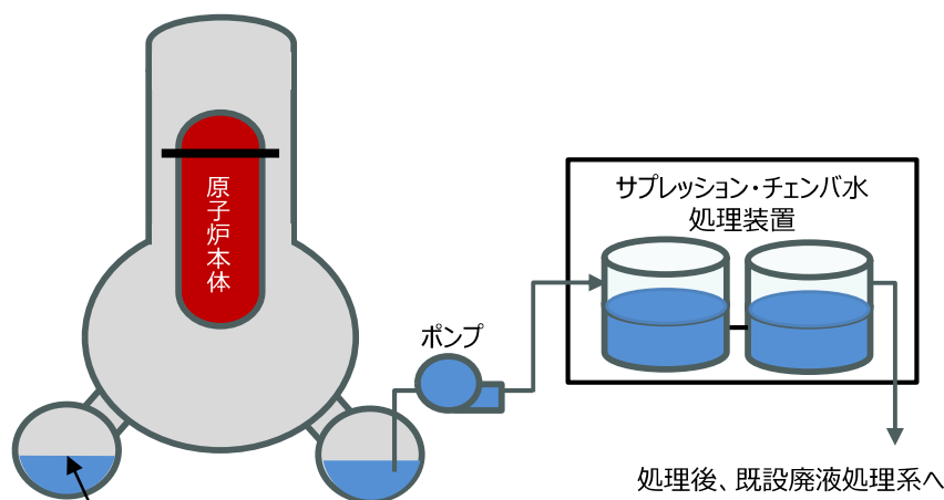
＜サプレッション・チェンバ水処理装置（概念図）＞
