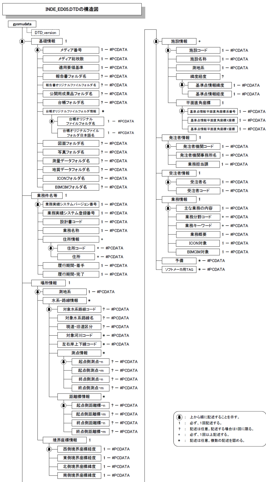
付図 1-1 業務管理ファイルの DTD の構造
