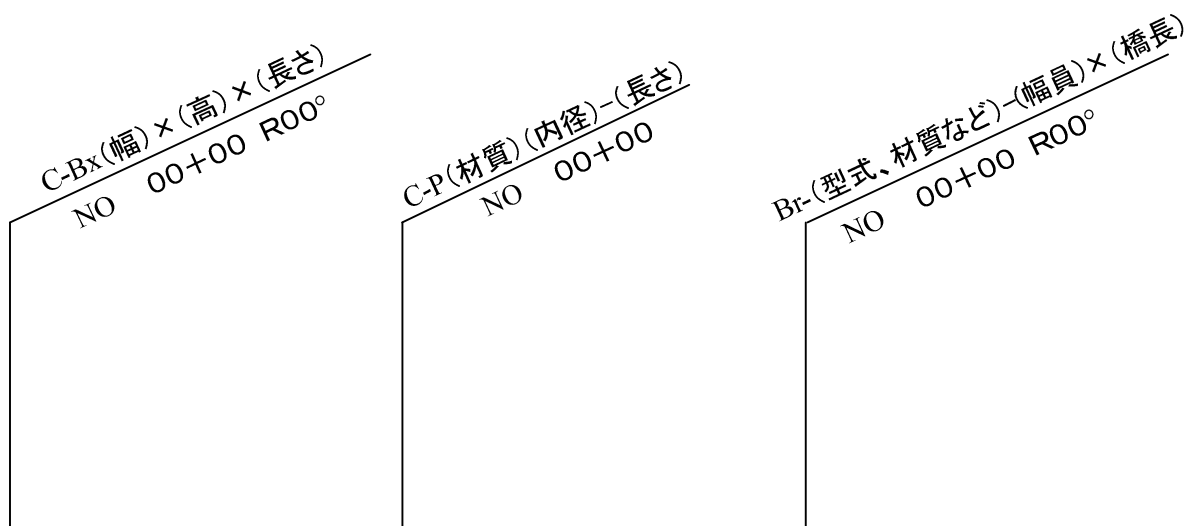
解説 図 2-3 横断構造物の旗上げ表現(例)
