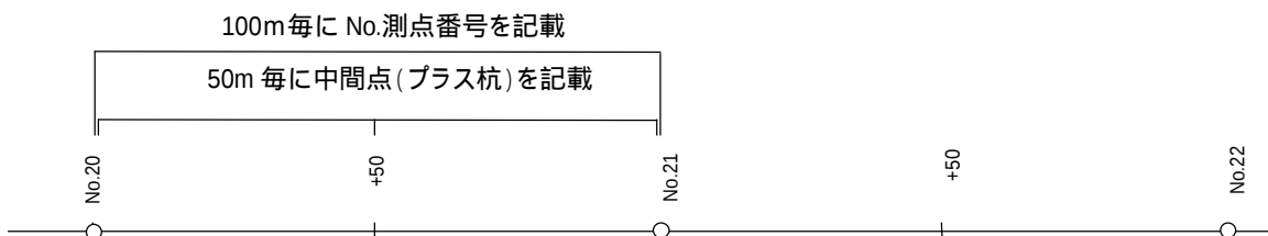
解説 図 6-1-1 平面線形の表現方法
