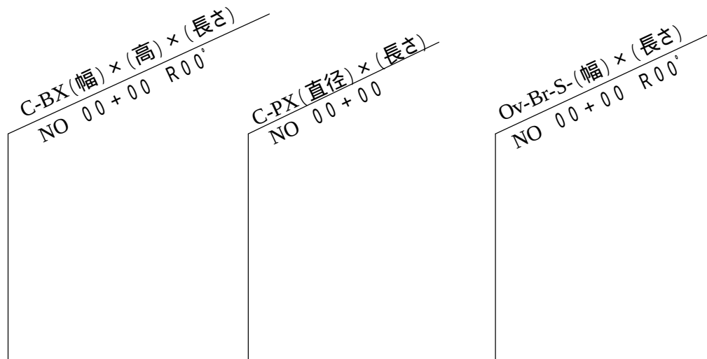
解説 図 6-6-2 横断構造物の旗上げ表現
