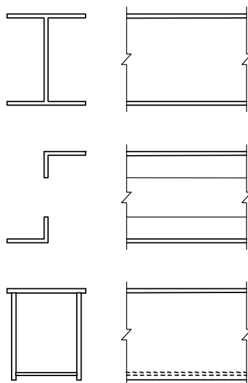
解説 図 6-7-1 形状の表示
