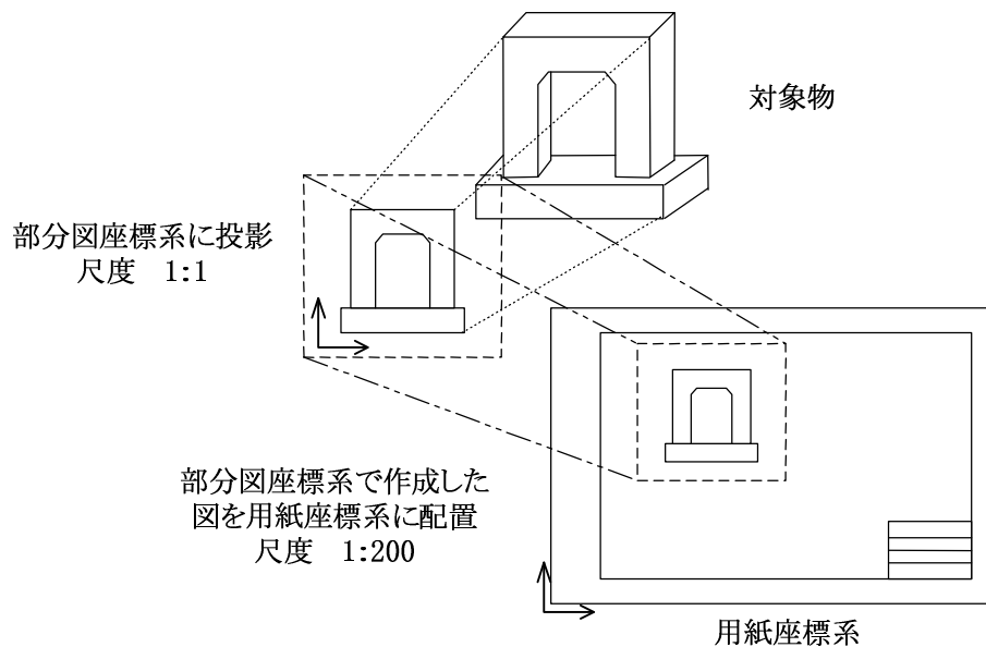
解説 図 1-7 用紙座標系と部分図座標系の関係
