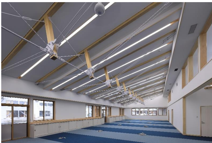
事務室(タイバートラス工法)
