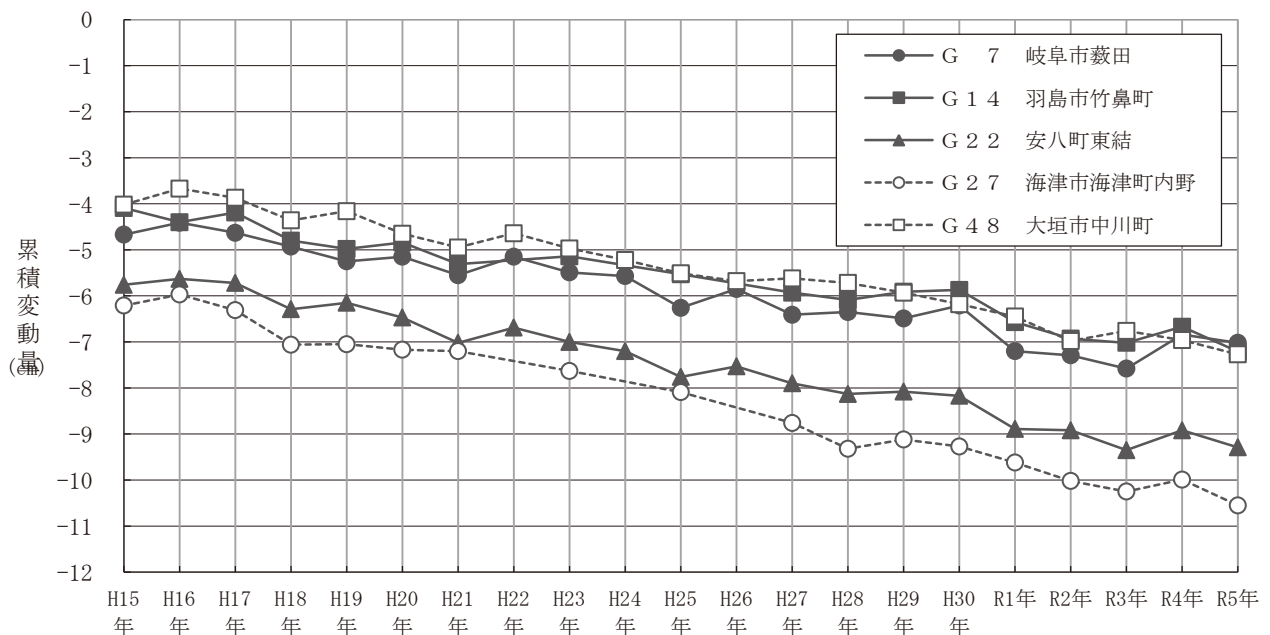
図2-4-21 主要水準点の累積変動量の経年変化
