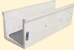
ECO-水路Ⅲ(ささゆり) 溶融スラグ(ささゆり) R5.2末で廃止 丸栄コンクリート工業(株) TEL 058-393-0221
