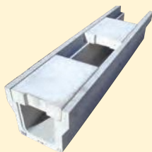
落ちふた式U形側溝・蓋・スタッド20(ノンスリップ模様) 溶融スラグ(中津川) 株式会社赤羽コンクリート TEL 0573-68-2632
