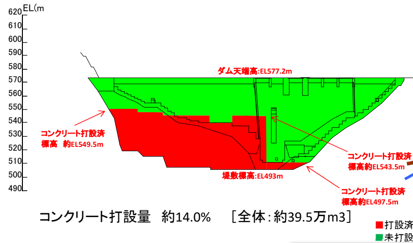
コンクリート打設進捗状況(R3.10末時点)
