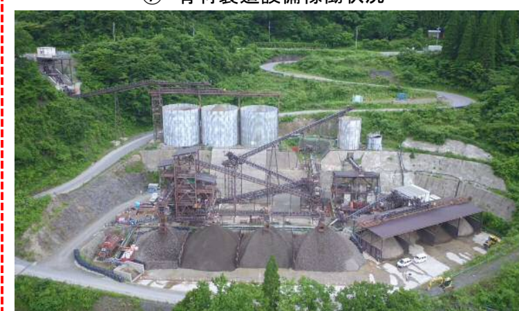
⑦ 骨材製造設備稼働状況
