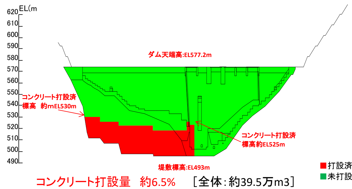
コンクリート打設進捗状況(R3.4末時点)
