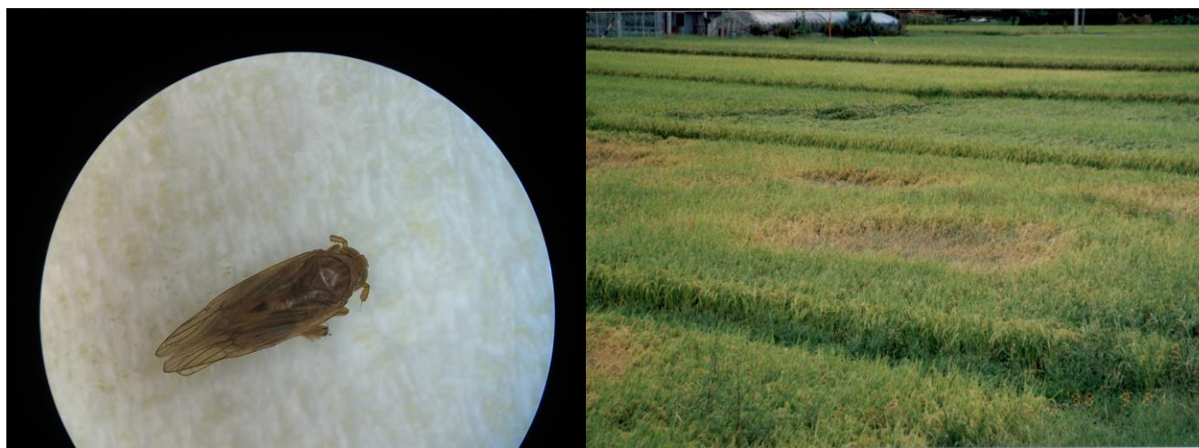
下呂市萩原町の予察灯に誘殺されたトビイロウンカ トビイロウンカによる坪枯れ被害(平成10年9月撮影)
