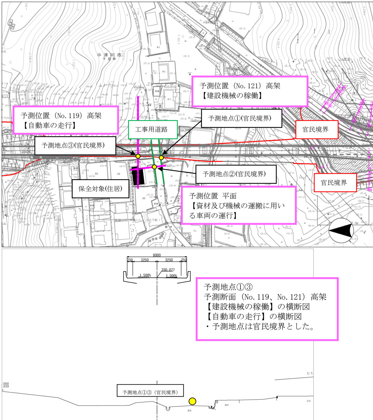
図 6.4-7(3)-1 予測位置図 (断面③)
