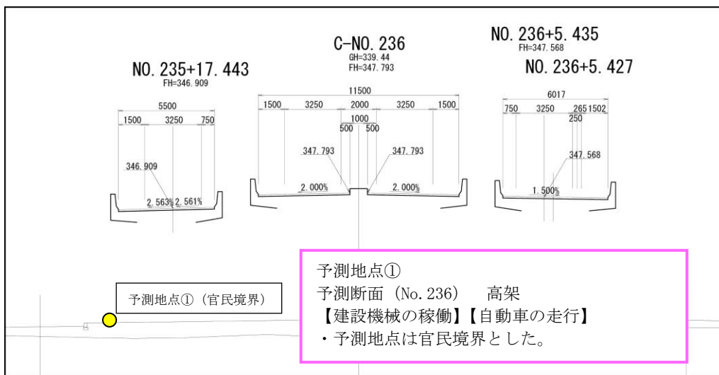
図 6.4-7(6)-1 予測位置図(断面⑥)
