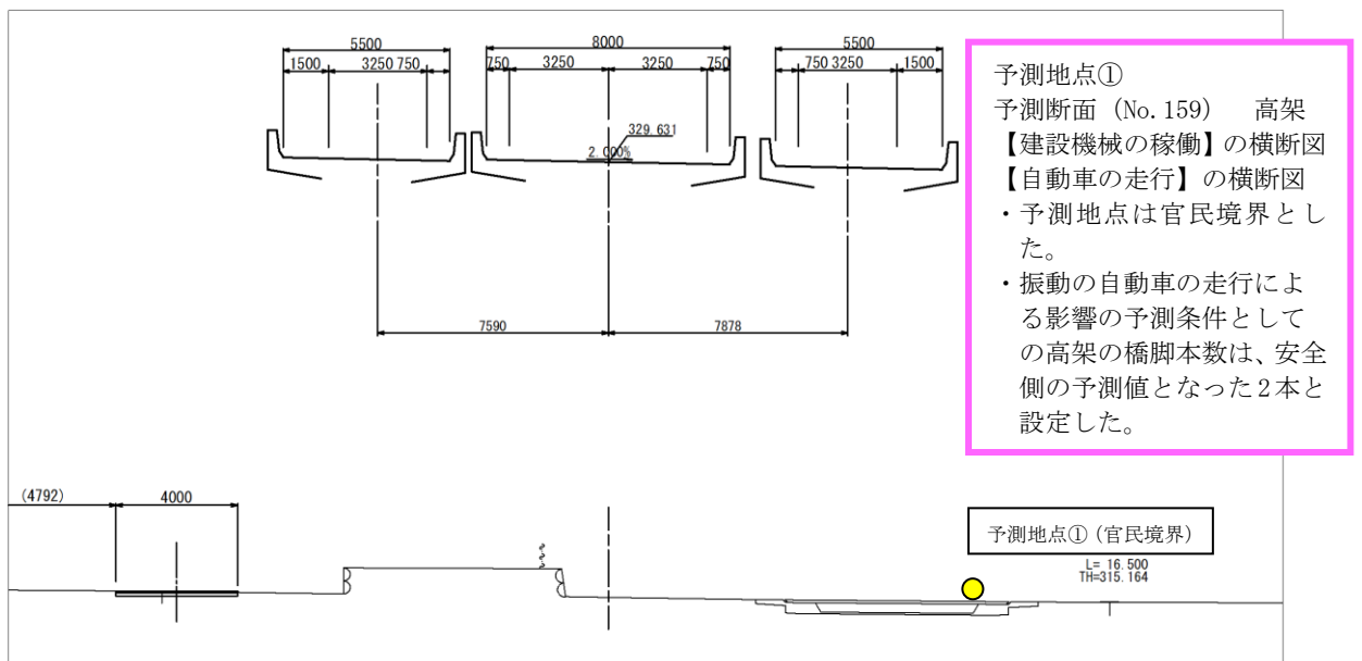
図 6.4-7(4)-1 予測位置図(断面④)
