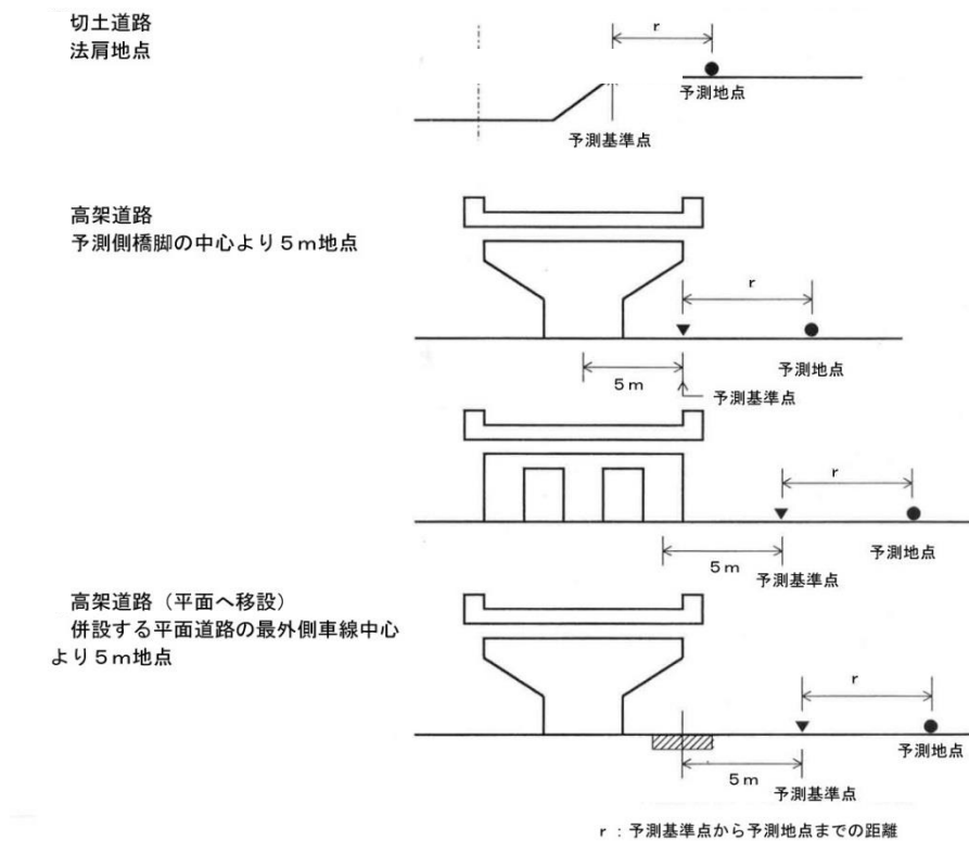
図 6.4-10 予測基準点の位置
