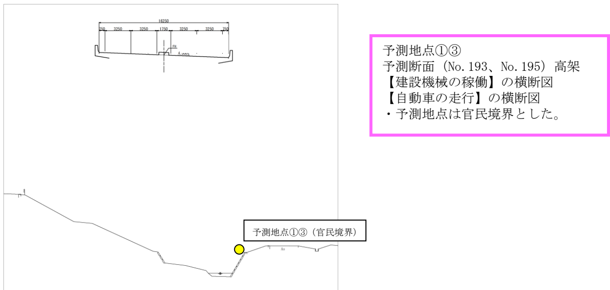
図 6.4-7(5)-1 予測位置図(断面⑤)
