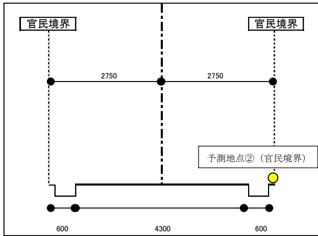
図 6.4-7(6)-2 予測位置図(断面⑥)
