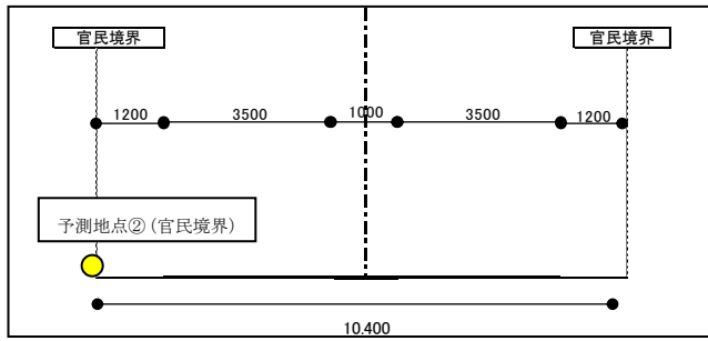
図 6.4-7(1)-2 予測位置図(断面②)
