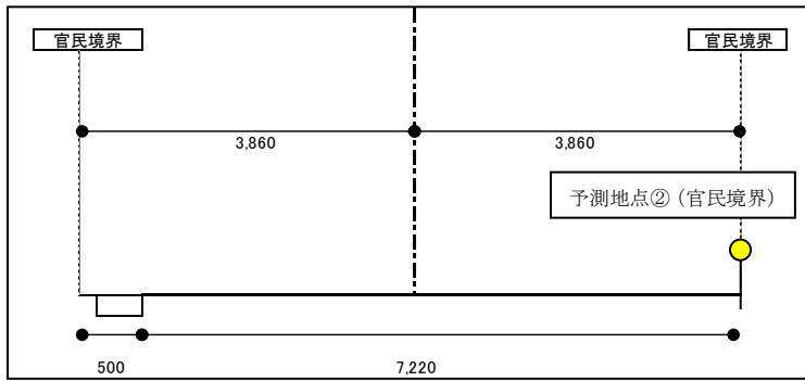
図 6.2-7(5)-2 予測位置図(断面⑤)
