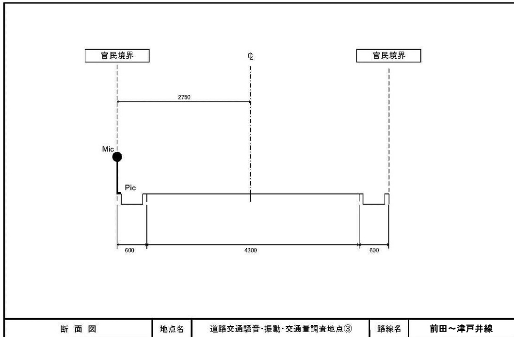
図 6.2-4 道路交通騒音調査 測定地点3・断面図
