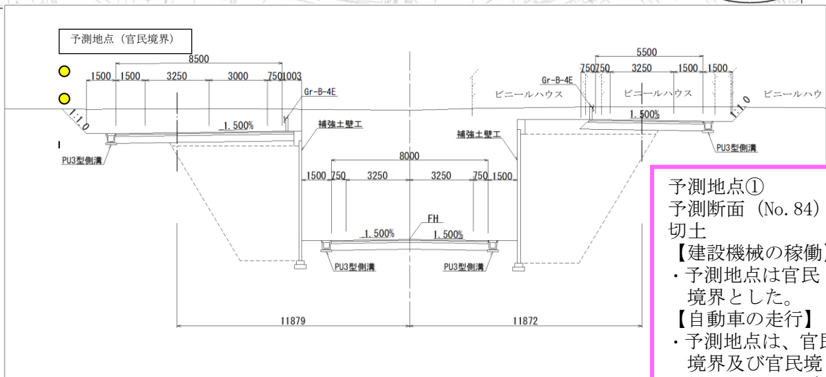
図 6.2-7(2)-1 予測位置図(断面②)
