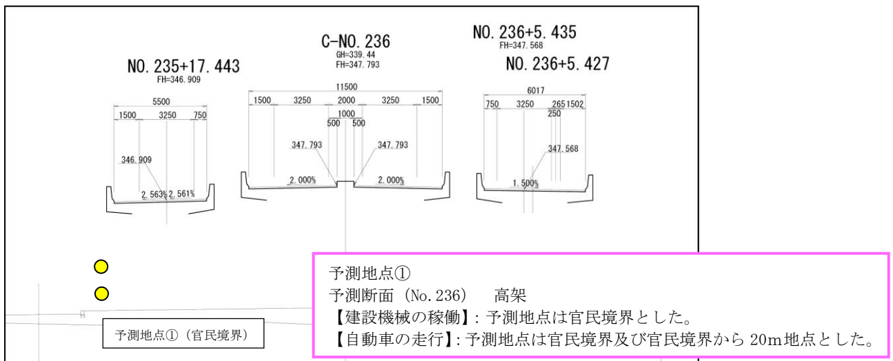
図 6.2-7(6)-1 予測位置図(断面⑥)
