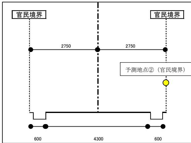
図 6.2-7(6)-2 予測位置図(断面⑥)
