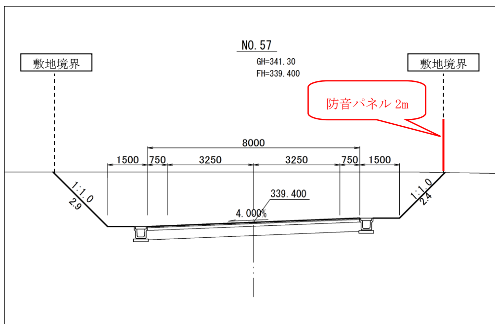
図 6.2-10 防音パネル設置イメージ(予測断面①切土)
