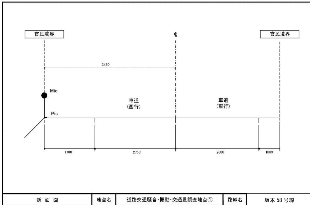
図 6.2-2 道路交通騒音調査 測定地点 1・断面図
