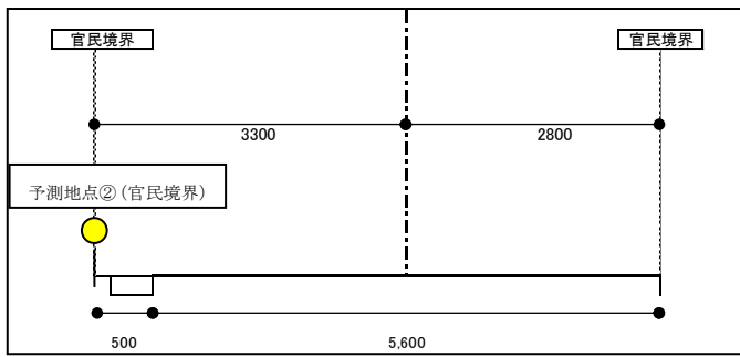
図 6.2-7(3)-2 予測位置図 (断面③)
