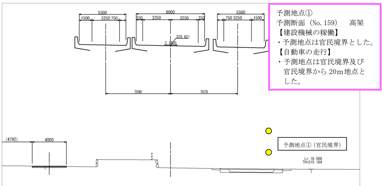
図 6.2-7(4)-1 予測位置図(断面④)
