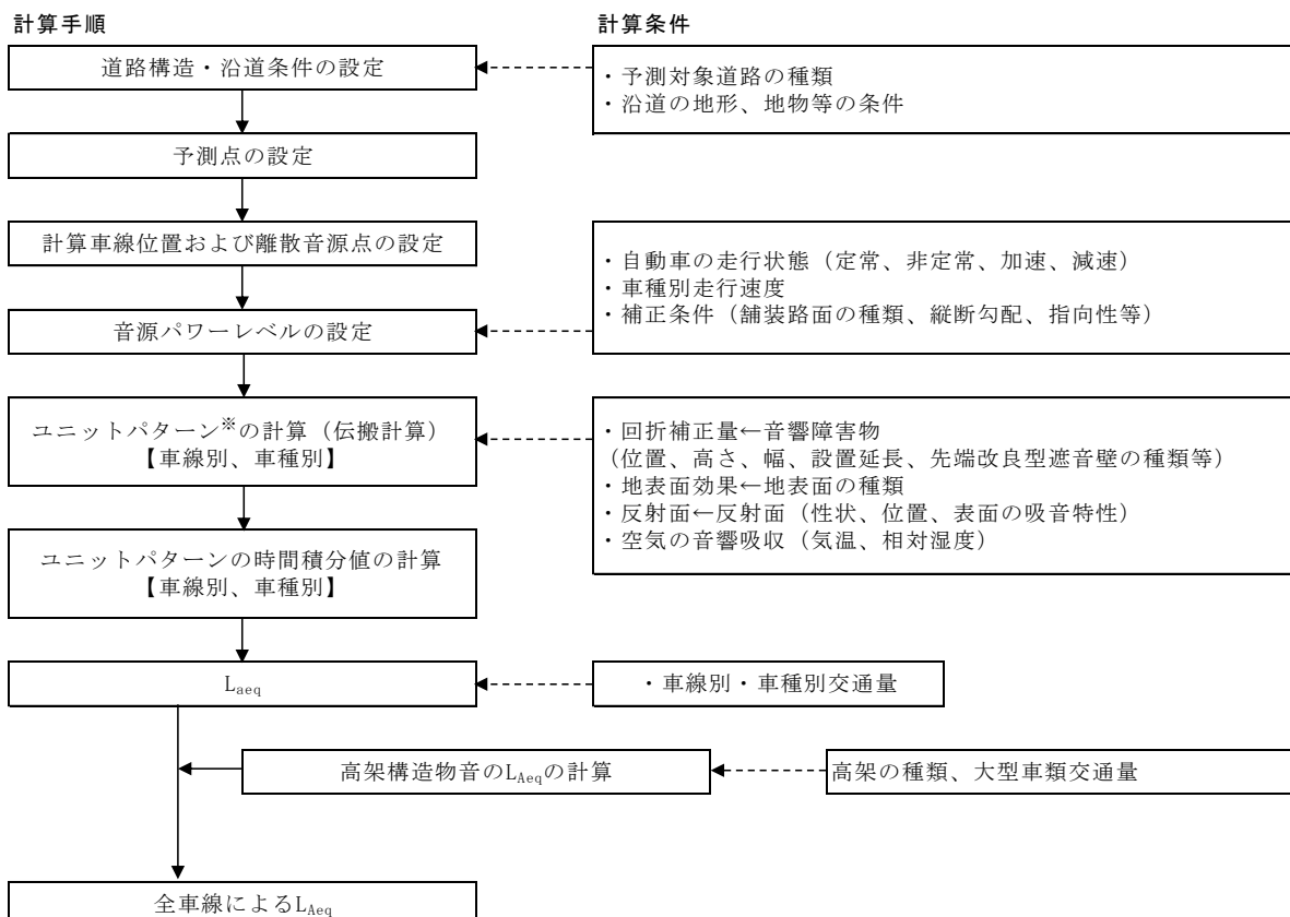
図 6.2-11 等価騒音レベル ( L_{Aeq} ) の予測方法
