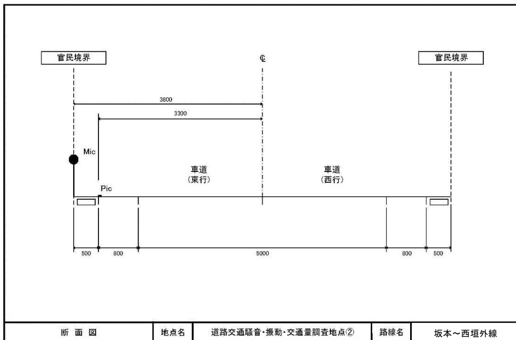
図 6.2-3 道路交通騒音調査 測定地点 2・断面図
