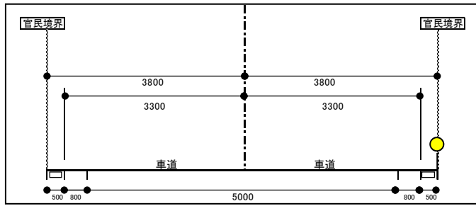
図 6.2-7(4)-2 予測位置図(断面④)
