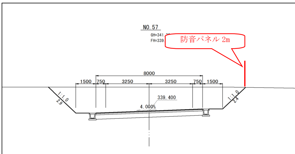
図 6.2-8 防音パネル設置イメージ(予測地点①（岩屋堂地区：切土部）)
