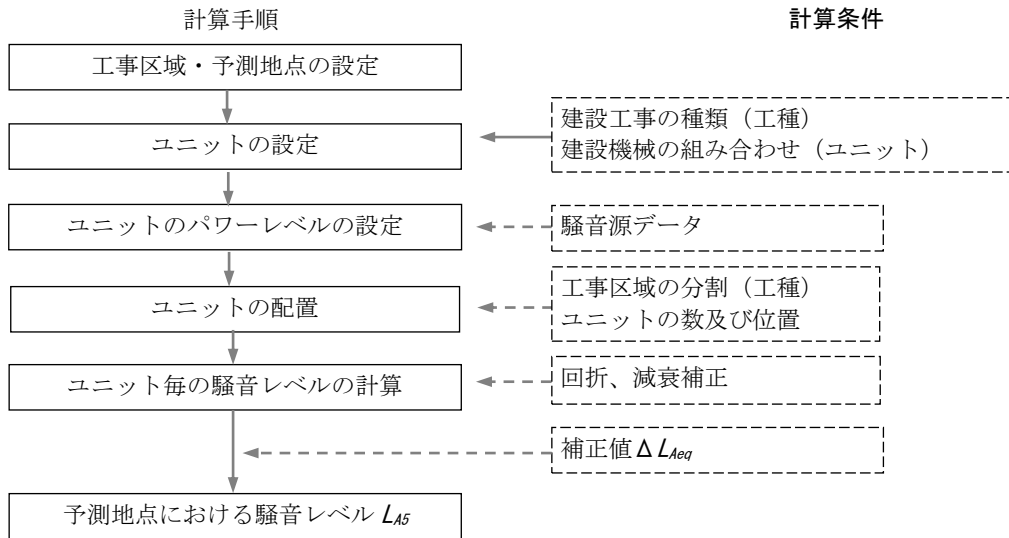
図 6.2-5 建設機械の稼働による騒音の予測手順
